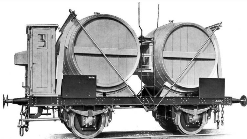
Zweiachsiger Faltwagen mit Bremse und Bremserhaus, mit 2 Fässern à 8500 Liter Inhalt, für Weintransport. Wagon-fut à 2 essieux avec frein et guérite à 2 futs, chaque fut d'une contenance de 8500 litres, pour le transport de vin. Wine reservoir truck with 2 axles, with screw brake and brakeman's cabin, with 2 barrels à 8500 l capacity. Vagones-foudres de dos ejes con freno de tornillo y garita, con 2 foudres a 8500 l de capacidad, para el transporte de vino.
