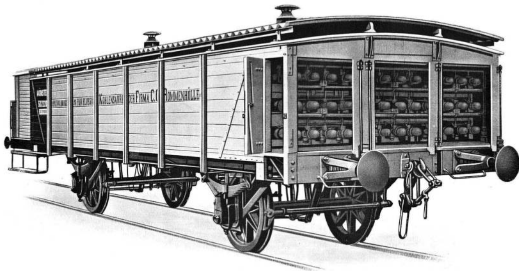
Bedeckter zweiachsiger Wagen mit Bremse, zum Transport von flüssiger Kohlensäure. Ladegewicht 6000 kg. Anzahl der Flaschen 36. Wagon couvert à 2 essieux avec frein, pour le transport de l'acide carbonique liquide. Chargement: 6000 kls. Nombre des tubes: 36. Covered truck with 2 axes, with screw brake, for transporting of liquiding carbonic-acid. Tonnage: 6000 kg. Number of steel-cylinders 36. Vagón cubierto de dos ejes con freno, para el transporte de ácido carbonico. Tonelaje: 6000 kg. Nombre de cilindros de acero: 36.
